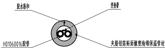
伴热保温局部视图
